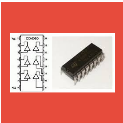
CD4050 / HEF4050 DIP
